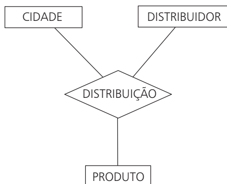
Figura 2.10 Relacionamento ternário.
