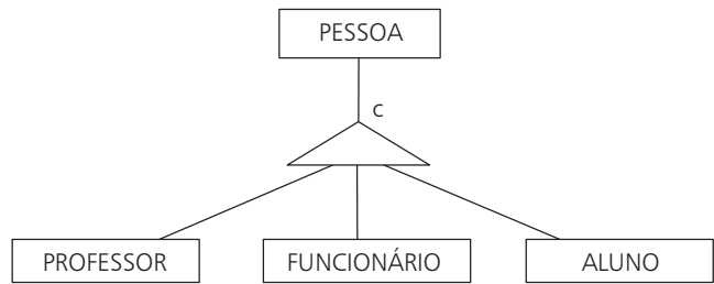
Figura 2.28 Generalização/especialização compartilhada.
