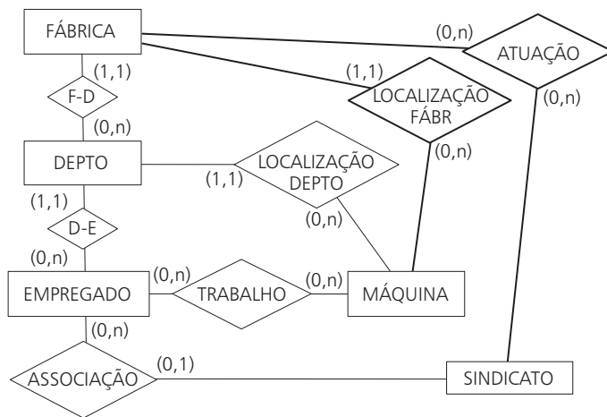
Figura 3.15 Relacionamentos redundantes.
